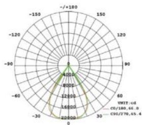
MODULE 60°
