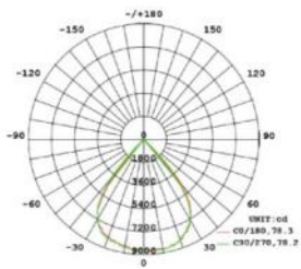
MODULE 90°
